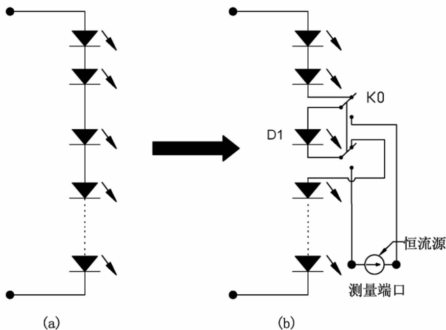
图 1 测量示意图
