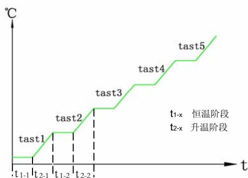
图 2 阶梯式控温曲线图
