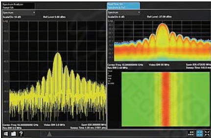
PXA/MXA 中的 RTSA 显示使用户可以查看 WLAN 和蓝牙的多猝发信号。
