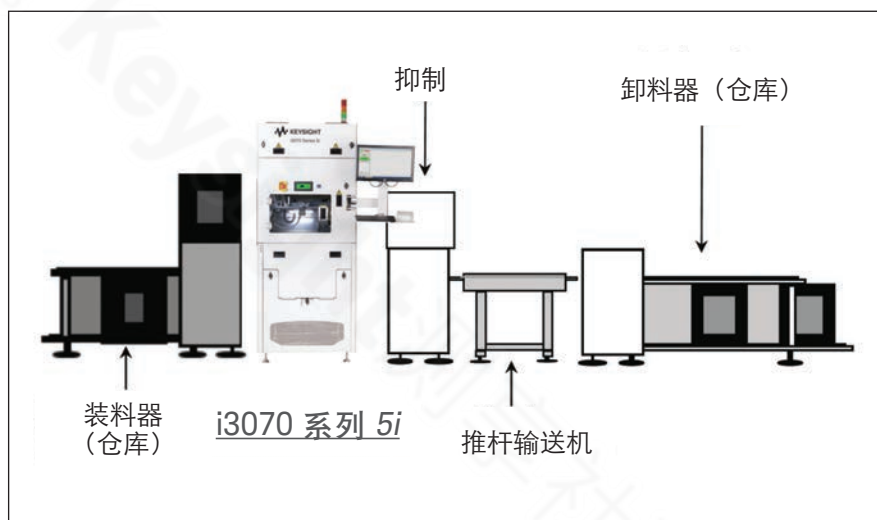
孤立模式部署实例
