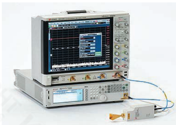
77/79 GHz 汽车雷达信号分析参考解决方案
