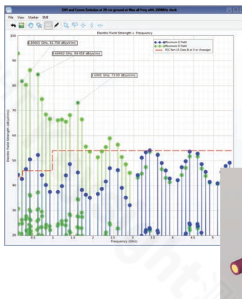
EMPro 提供的电磁仿真器能预测电子元件和电缆的电磁辐射水平
