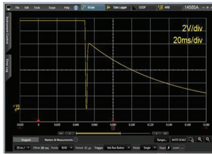
ISO 7637-2: 5.6.2 采用 APS 和 14585A 测试脉冲 2b 电机瞬态生成
