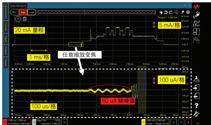
图 4. 放大后的图 3 中休眠模式下的波形。
